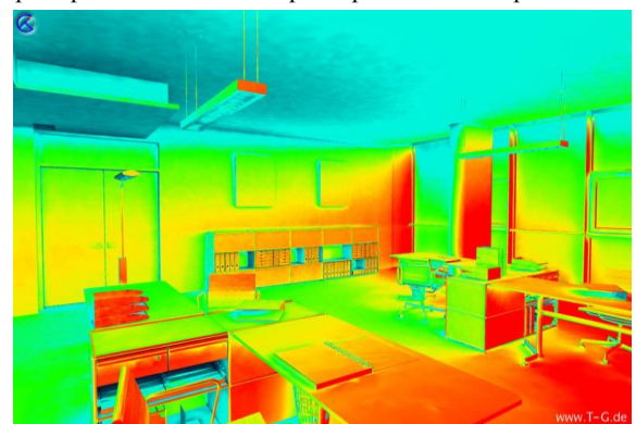
Рис. 1. Распределение освещенности, представленное световой картой.
